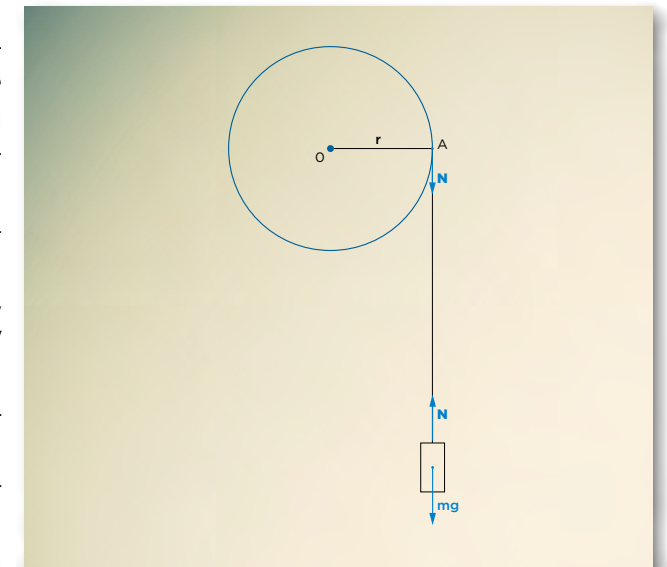
Rys. 1.3. Obrót walca
