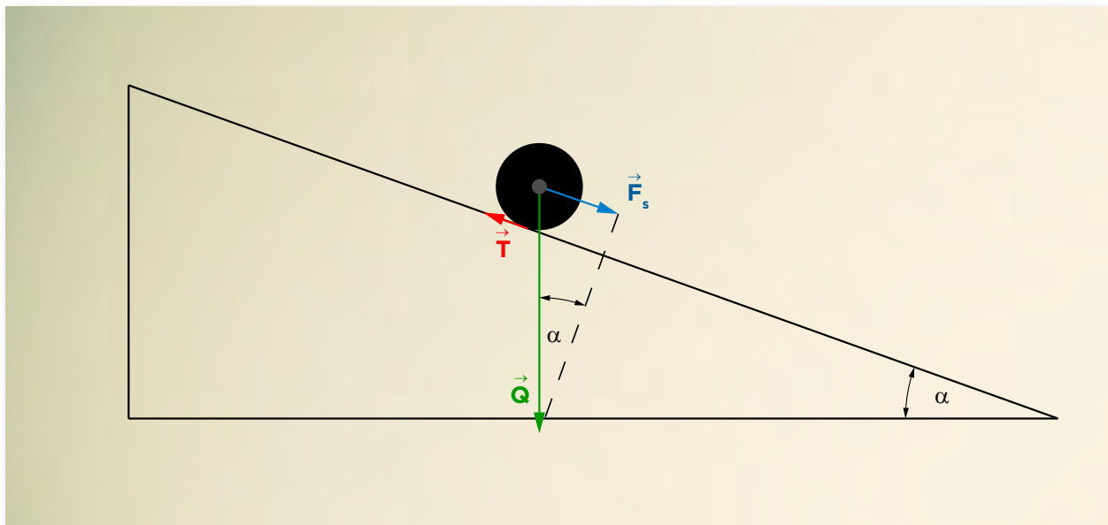
Rys. 3.3. Rozkład sił.
