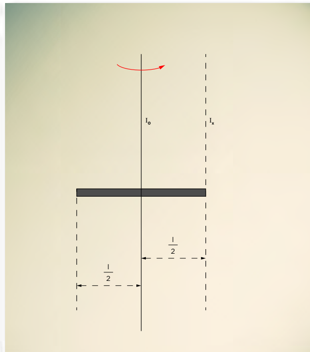
Rys. 1.6. I_0, I_x – momenty bezwładności pręta względem dwóch równoległych osi.
