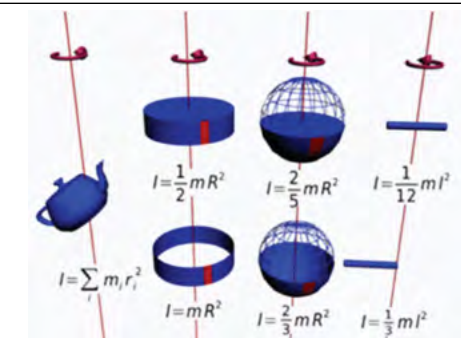
Rys. 1.4. Bryła sztywna
