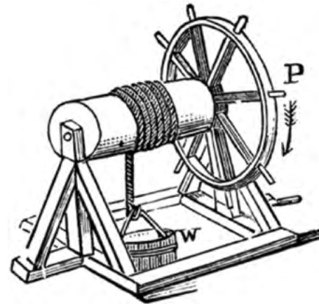
Rys. 3.1. Rycina przedstawiająca kołowrót ( http://pl.wikipedia.org/wiki/Plik:Whe-elaxle_quackenbos.gif )
